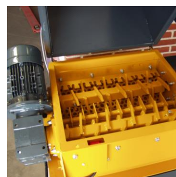
Twee getande assen zorgen voor een efficiënte vermaling.
